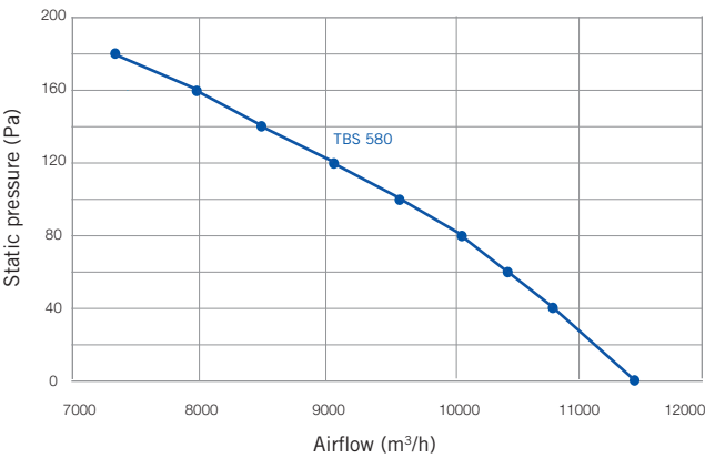
FAN CURVE
